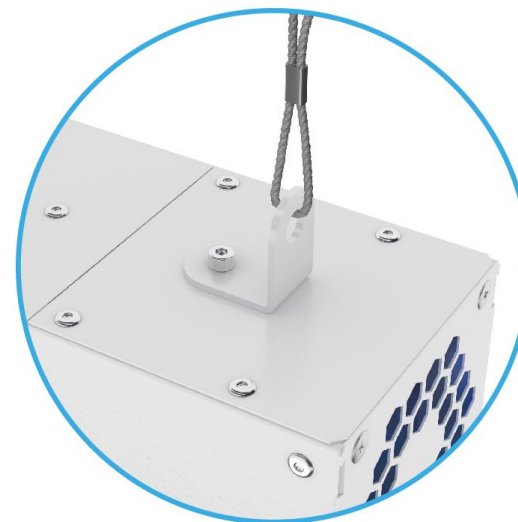
ПОДВЕСНОЙ МОНТАЖ
